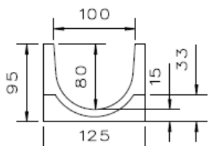
Vaterstück Masstab 1:4
