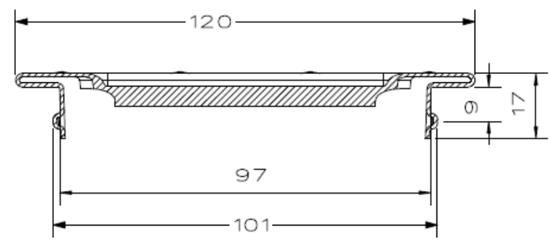
A-A Masstab 1:1
