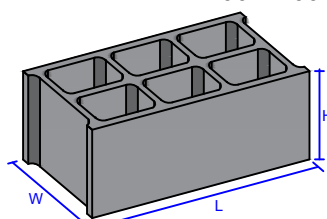
Bloco de Betão 500 x 200 x 200
