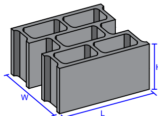
Bloco de Betão 400 x 200 x 270
